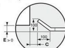
Détail 1 - Vue de dessus Detail 1 - Top view
