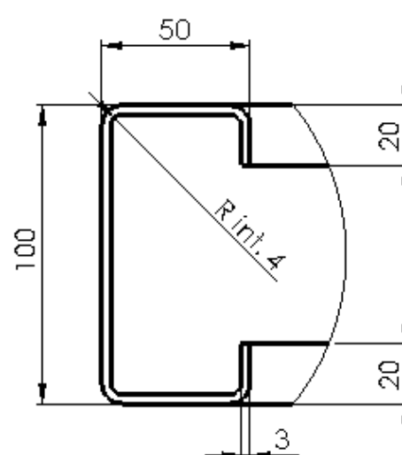
DÉTAIL A ECHELLE 1 : 2
