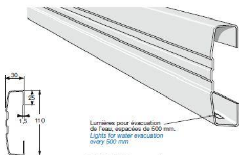
31.10169 ← 7 m → 31.10170 ← 5 m → 31.10171 ← 3,2 m → Profil protection latérale, acier galvanisé .
