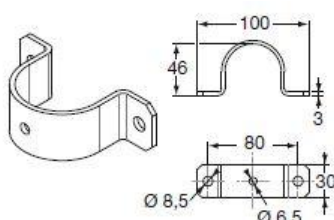
31.09054 \frac{Kg}{\Delta} 0,110 Collier de bridage acier galvanisé (sans visserie).
