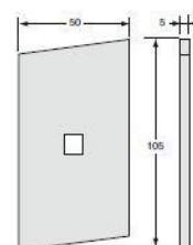
31.10177 \frac{Kg}{\Delta} 0,170 Plaque de fixation pour 31.10169/170/171, acier zingué
