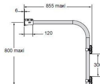
31.09051 \frac{Kg}{\Delta} 6,000 Tube cintré Ø 48,3, acier galvanisé .
