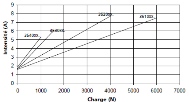
Intensité / Charge - moteur 12V
