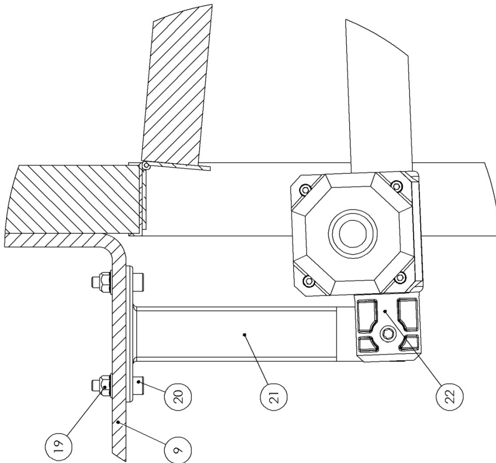
DÉTAIL B ECHELLE 1 : 2
