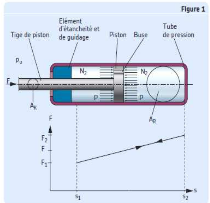
Schéma du ressort à gaz
