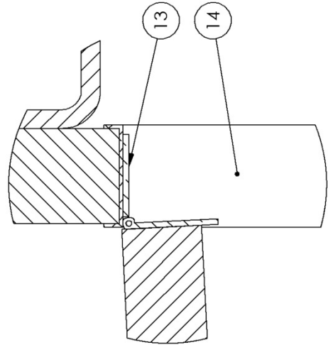
DÉTAIL G ECHELLE 1 : 2
