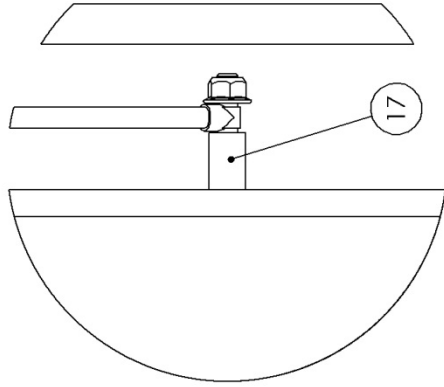
DÉTAIL D ECHELLE 1 : 2
